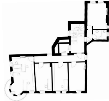
4. Obergeschoss
